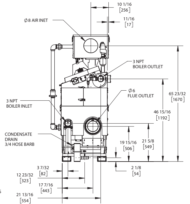
REAR VIEW ASUB-00051_D
