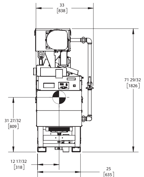
FRONT VIEW ASUB-00051_D
