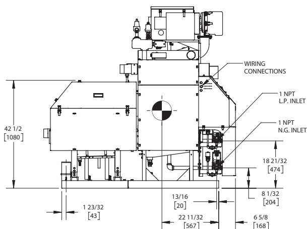
SIDE VIEW ASUB-00056_B
