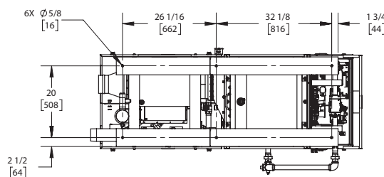
BOTTOM VIEW ASUB-00056_B
