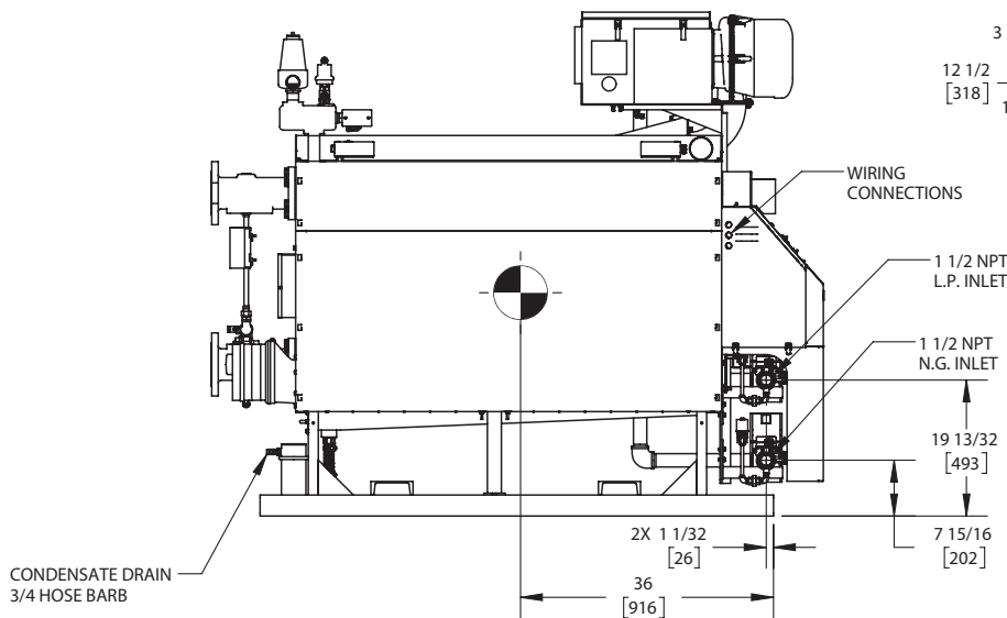
SIDE VIEW ASUB-26_E
