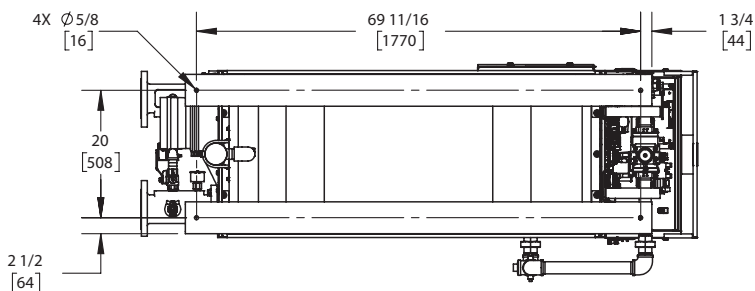
BOTTOM VIEW ASUB-26_E
