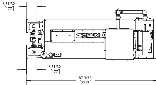
TOP VIEW ASUB-26_E
