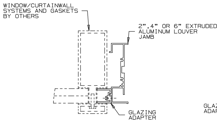
JAMB DETAIL
