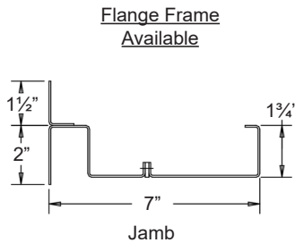
Jamb
